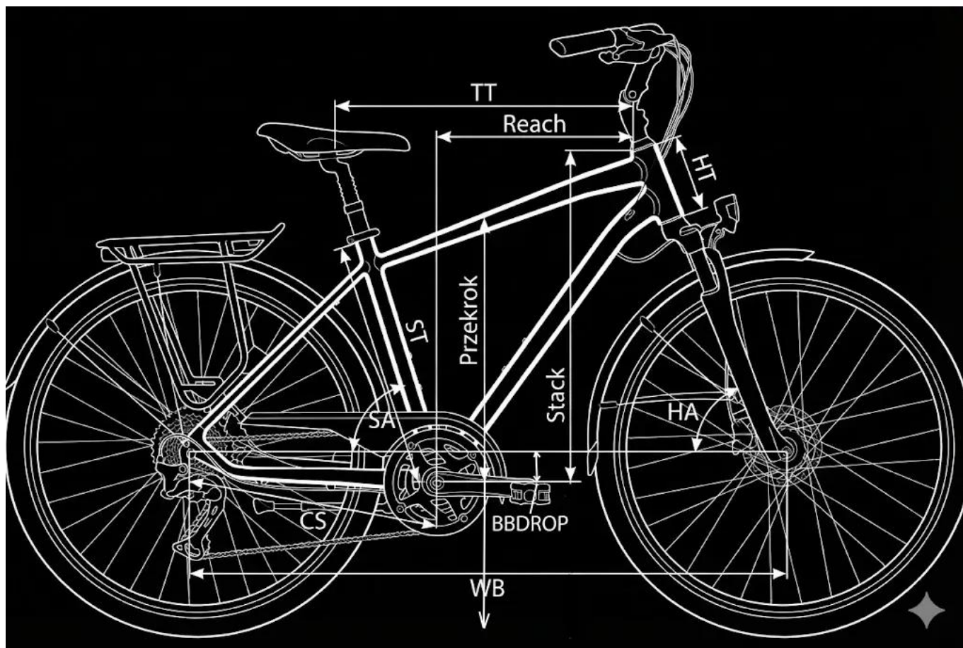
Geometria ramy trekkingowej BERG TR 5.0
