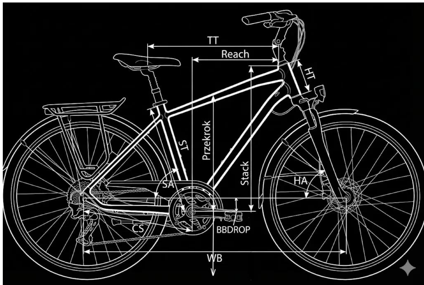
Geometria ramy BERG TR 3.0
