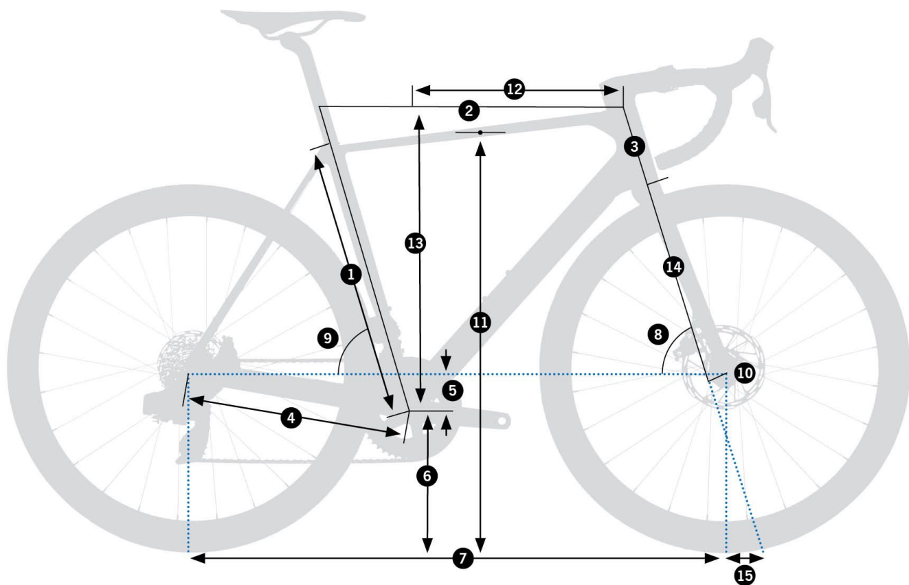
Orbea Orca M30i 2026 – schemat geometrii ramy (źródło: OBOOK 2026)
