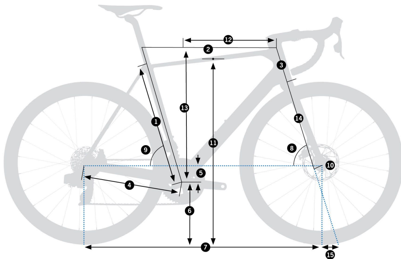
Orbea Orca M21eTEAM 2026 - schemat geometrii ramy (źródło: OBOOK 2026)
