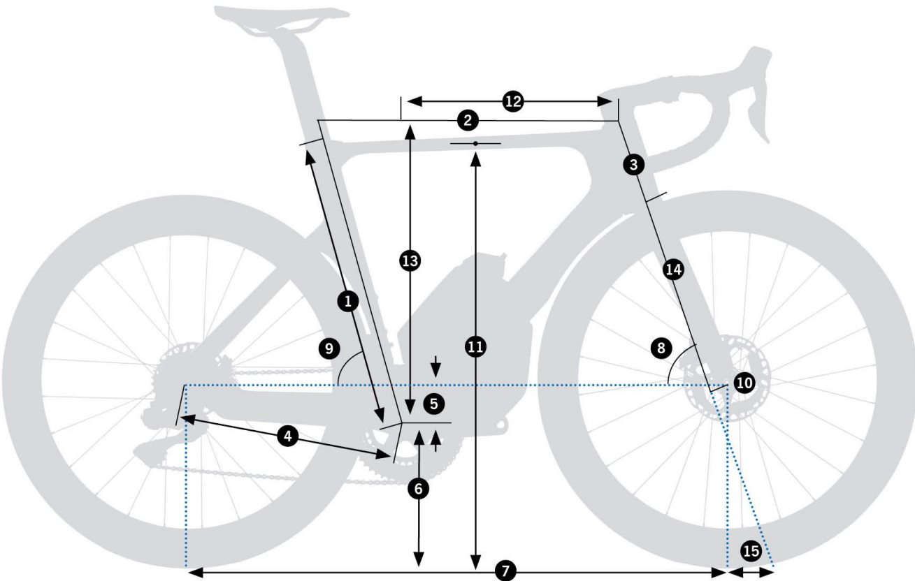
Orbea Orca Aero M21eLTD 2026 - schemat geometrii ramy (źródło: OBOOK 2026)
