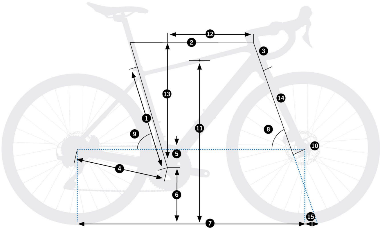
Orbea Avant H45 1x 2026 – schemat geometrii ramy (źródło: OBOOK 2026)
