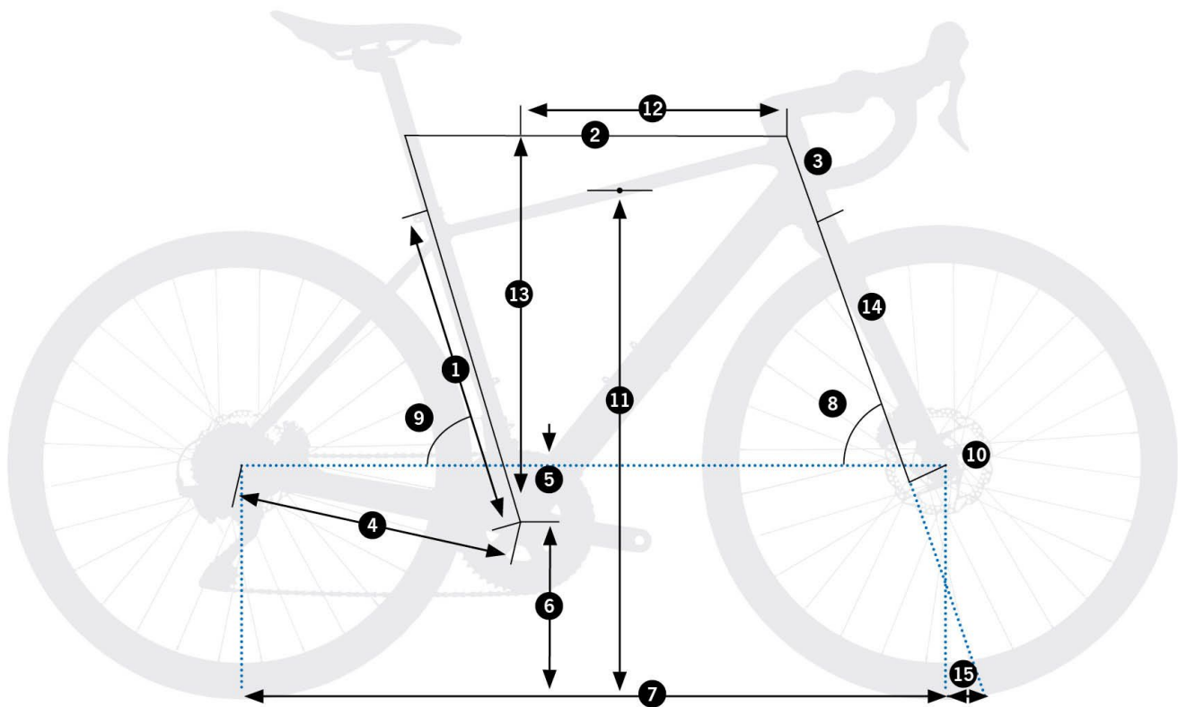
Orbea Avant H40 2026 – schemat geometrii ramy (źródło: OBOOK 2026)
