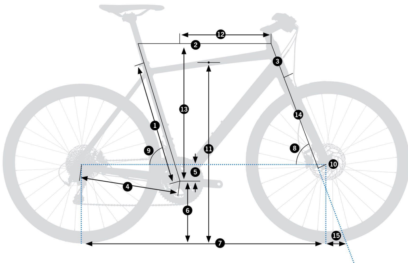
Schemat pomiarowy geometrii Orbea Vector 25 EQ 2026
