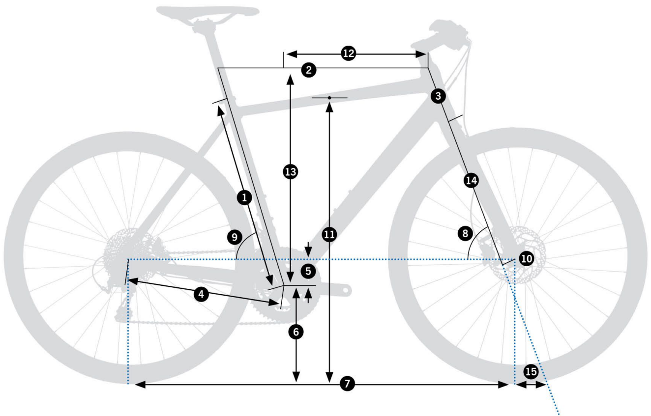
Schemat pomiarowy geometrii Orbea Vector 20 2026
