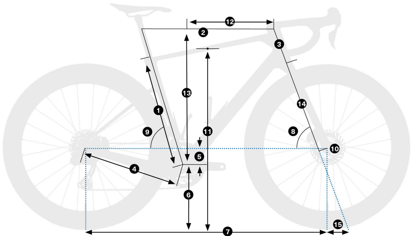
Orbea Terra Race M11eLTD 1X 2026 - schemat geometrii ramy (źródło: OBOOK 2026)
