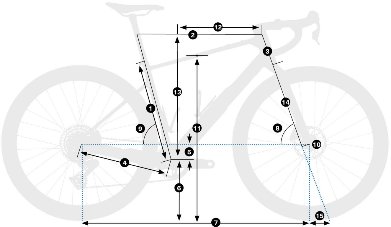
Orbea Terra M30TEAM 2026 - schemat geometrii ramy (źródło: OBOOK 2026)
