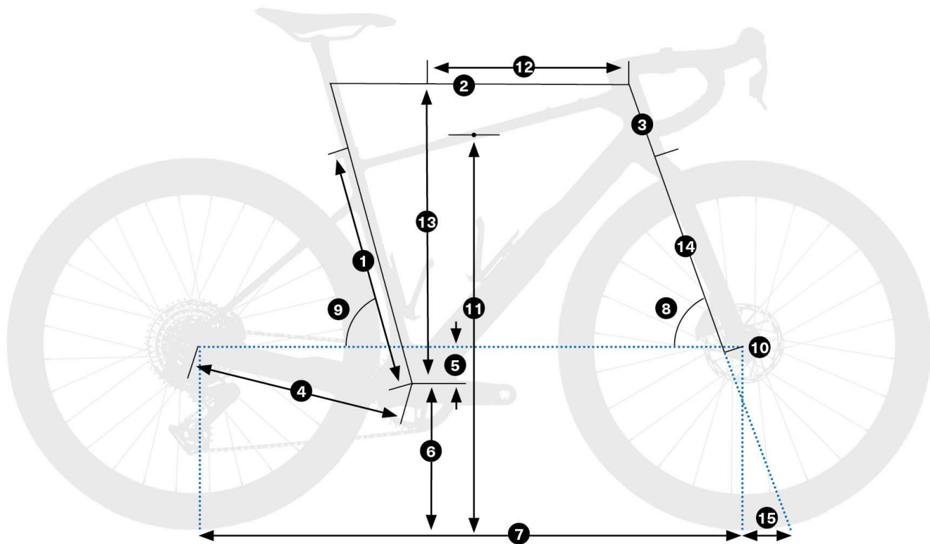
Orbea Terra M30TEAM 1X 2026 – schemat geometrii ramy (źródło: OBOOK 2026)
