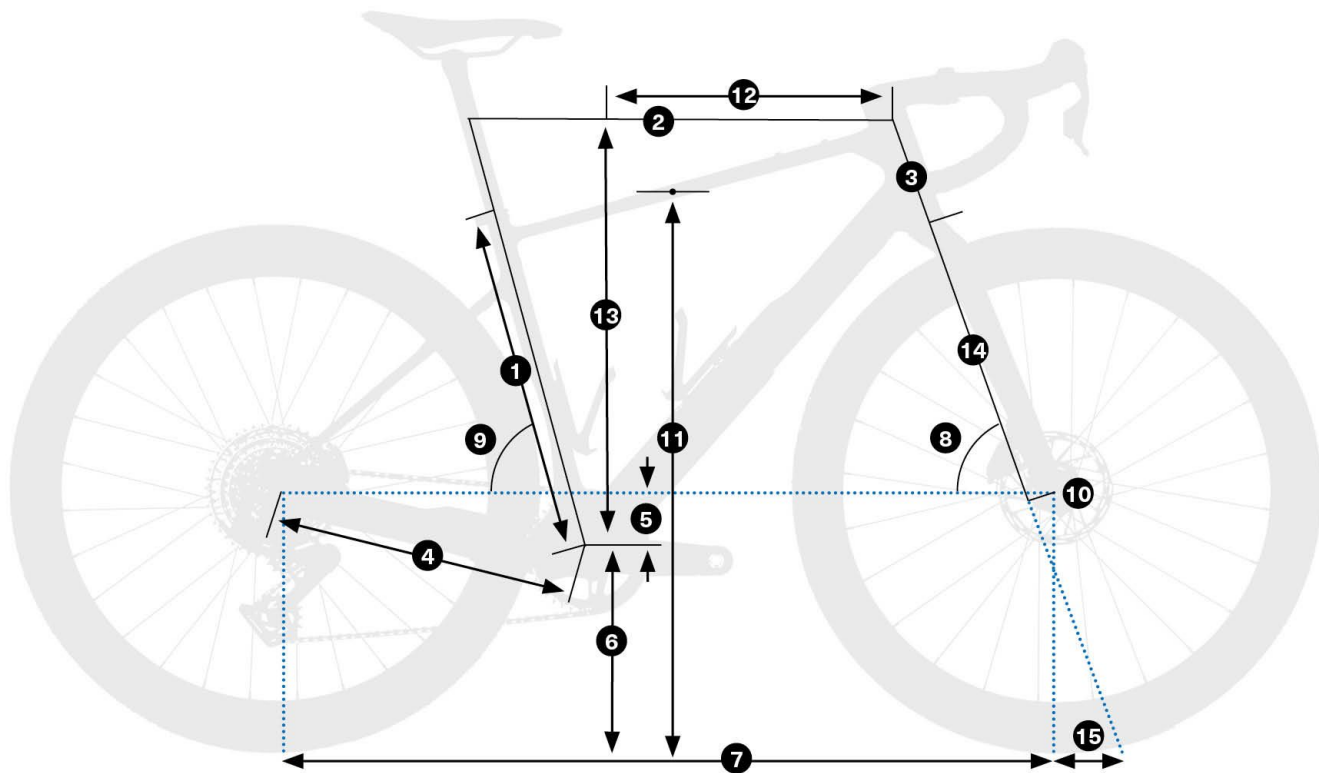
Orbea Terra M21eTEAM 1X 2026 – schemat geometrii ramy (źródło: OBOOK 2026)
