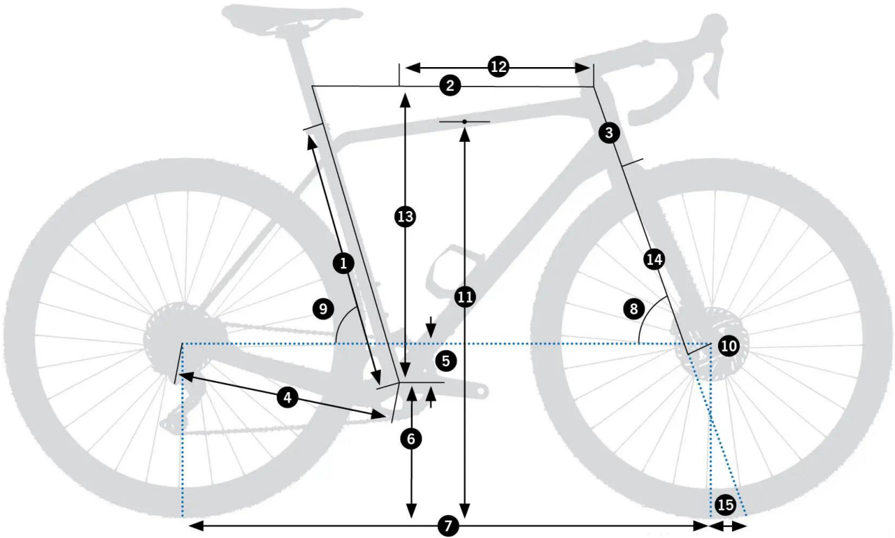
Orbea Terra H30 1x - schemat geometrii ramy
