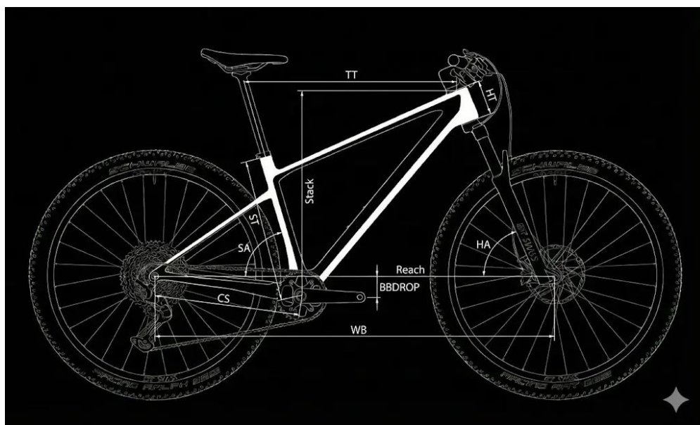
Rysunek techniczny – geometria ramy serii XP Carbon
