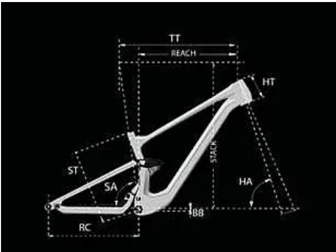
Schemat pomiarowy geometrii Lapierre Zesty CF
