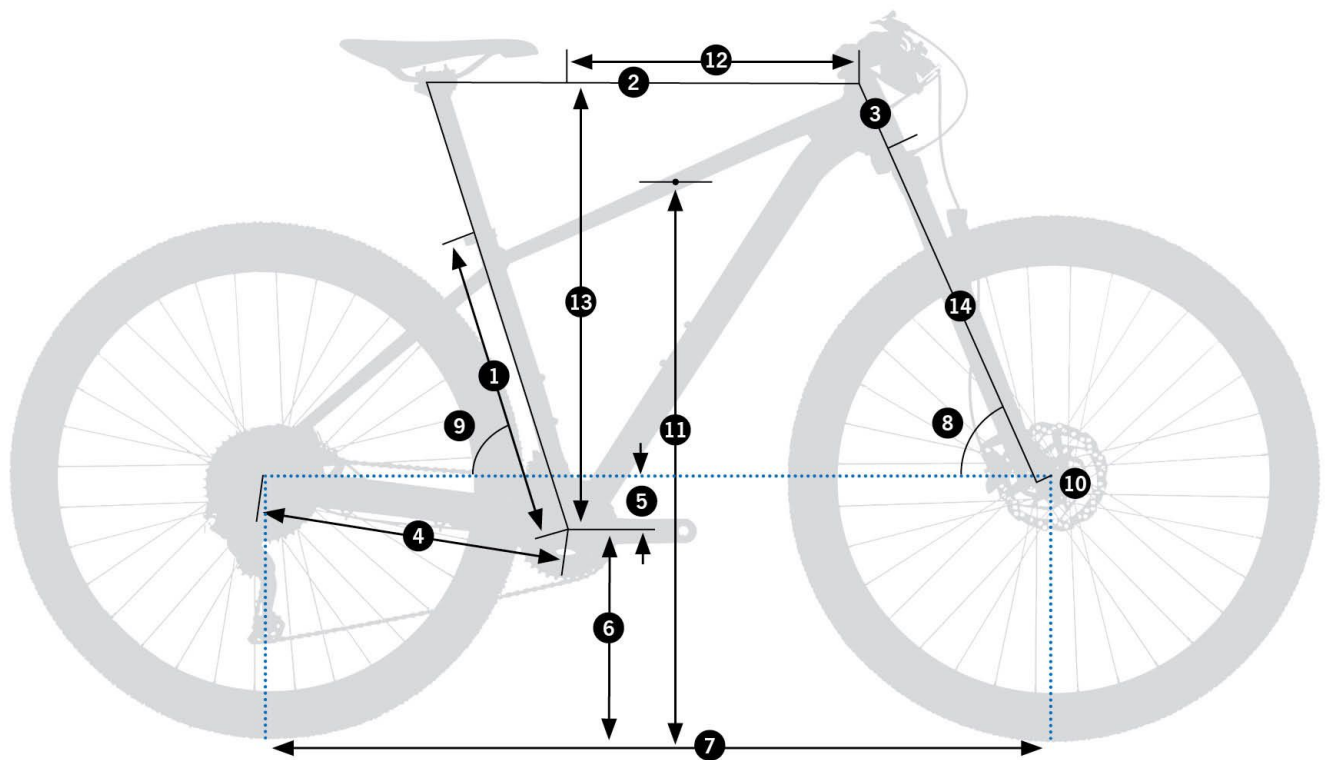
Orbea Onna 30 – schemat geometrii ramy
