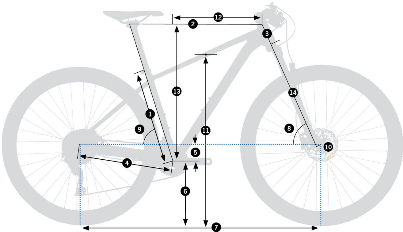
Orbea Onna 50 – schemat geometrii ramy
