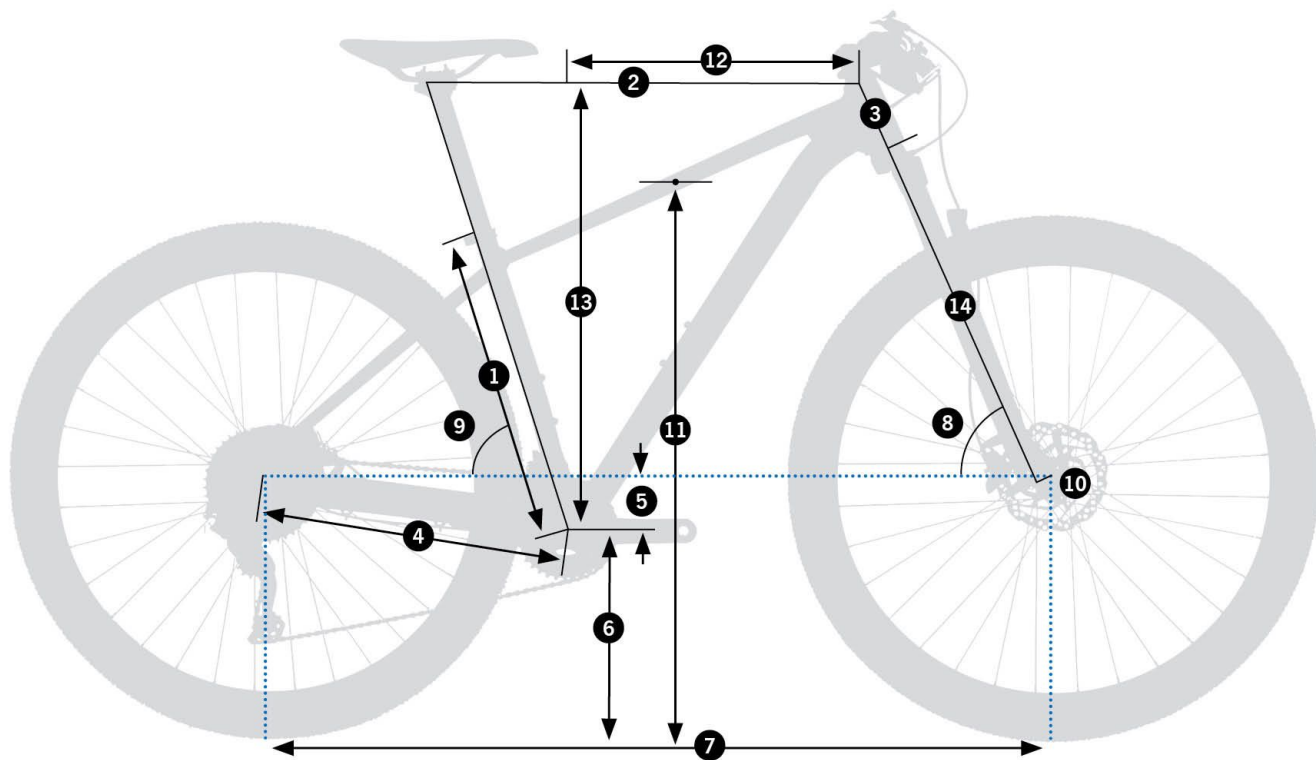
Orbea Onna 40 - schemat geometrii ramy
