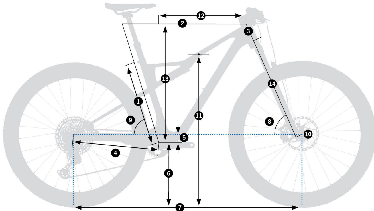
Orbea Oiz M-TEAM AXS 2026 – schemat geometrii ramy (źródło: Orbea)
