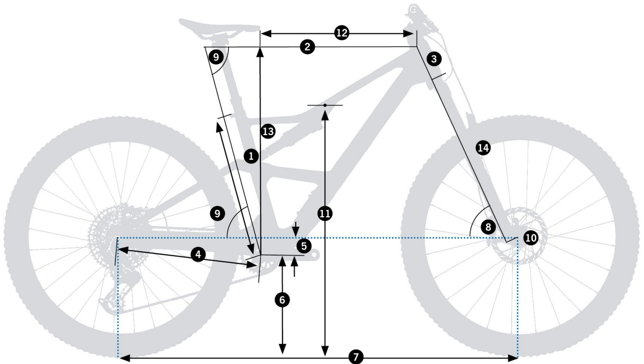
Orbea Occam SL Hydro 2026 – schemat geometrii ramy (źródło: Orbea)
