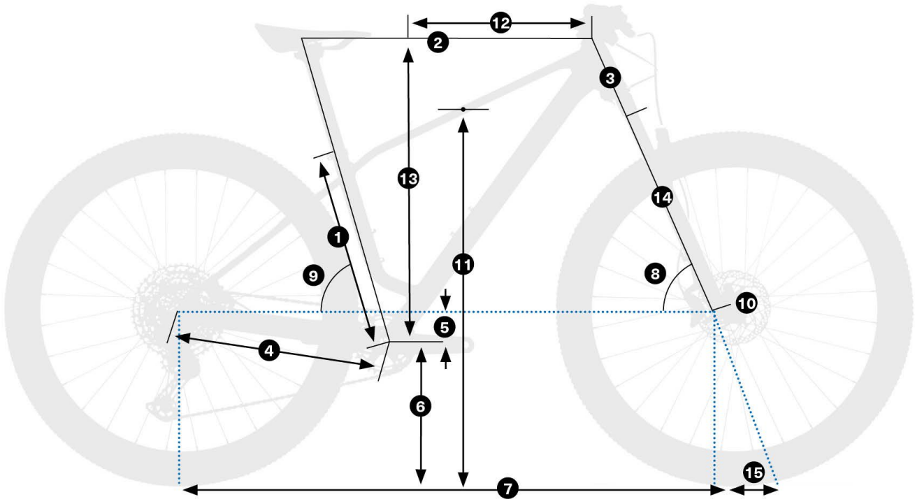
Orbea Alma H30 2026 - schemat geometrii ramy
