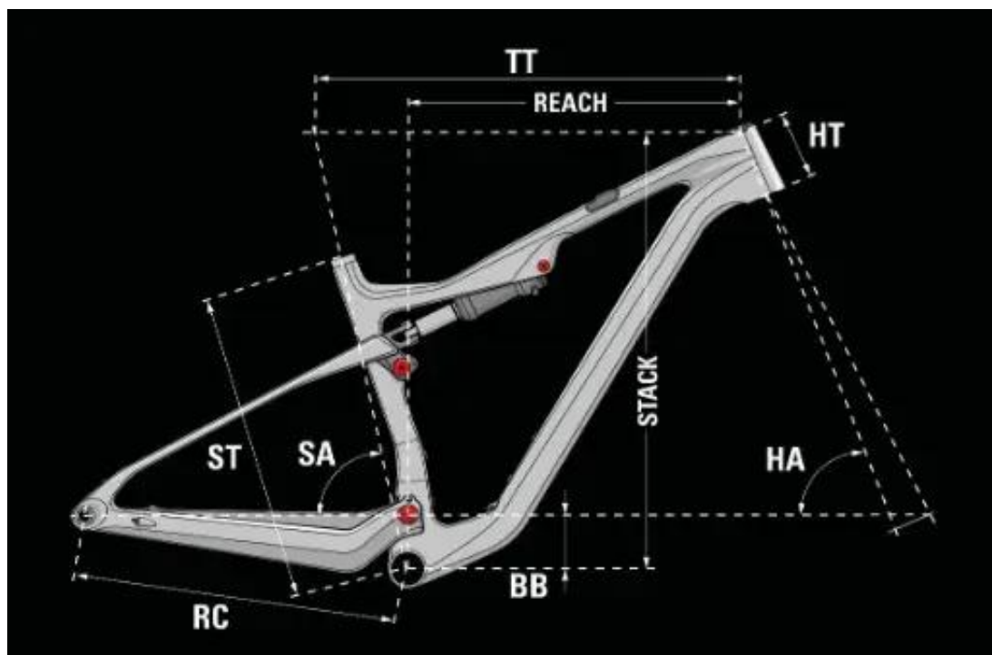
Schemat pomiarowy
