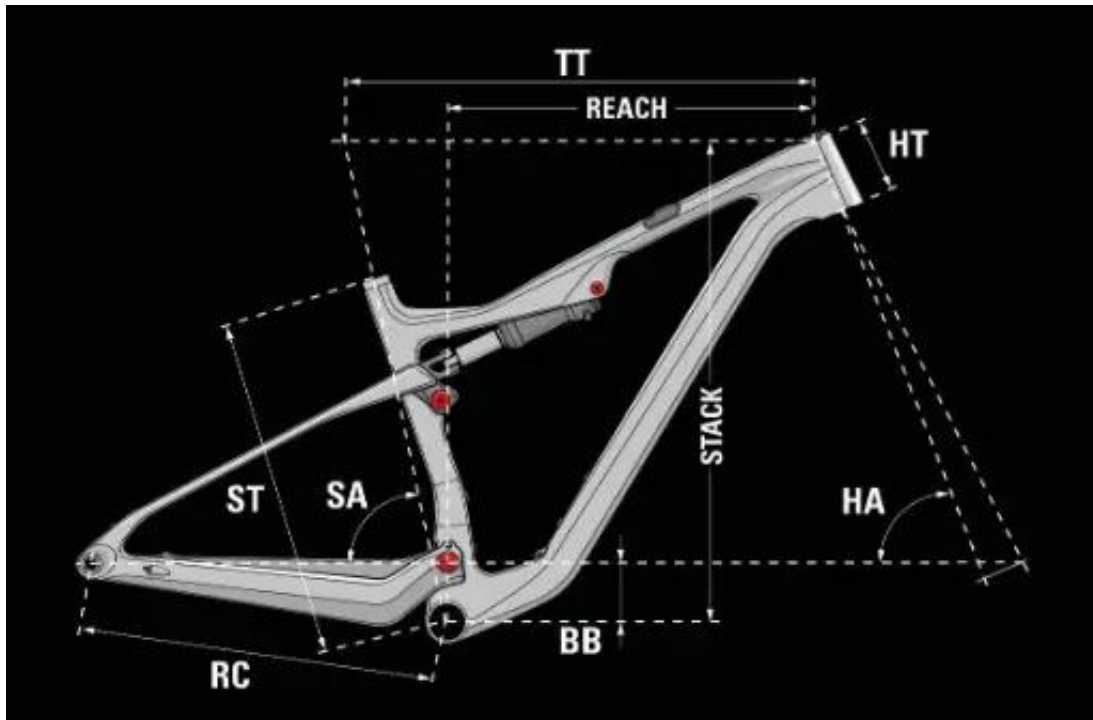
Schemat pomiarowy
