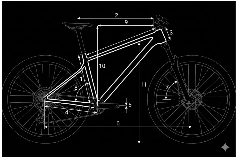
Rysunek techniczny – geometria ramy Lector (SuperFit)
