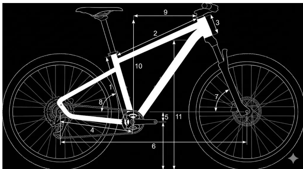
Rysunek techniczny - geometria Kato (Size Split)
