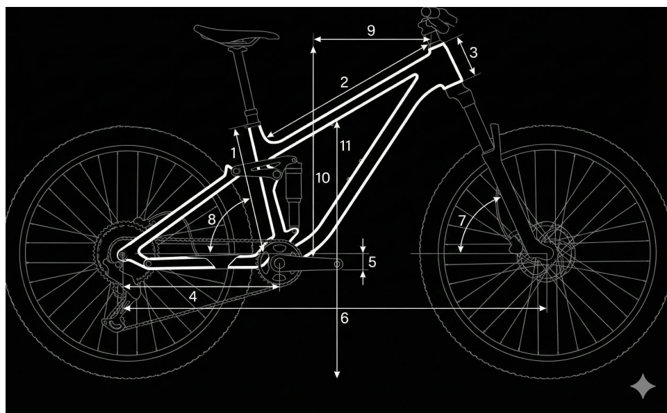
Rysunek techniczny - geometria Kato FS (Size Split)
