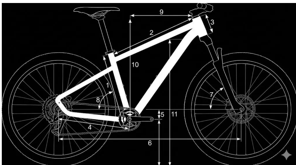
Rysunek techniczny - geometria ramy Kato (Size Split)
