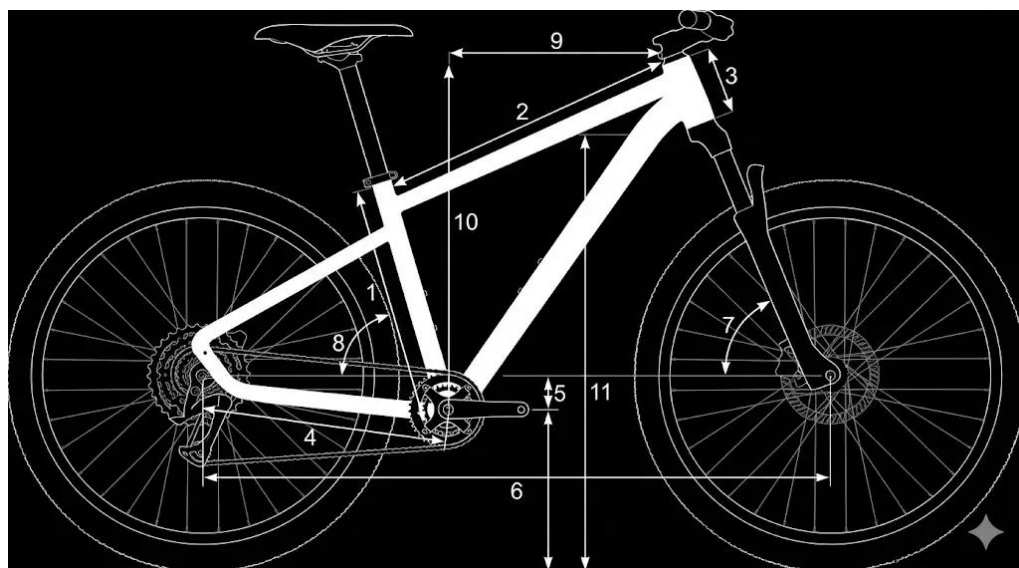
Rysunek techniczny - geometria Kato (Size Split)
