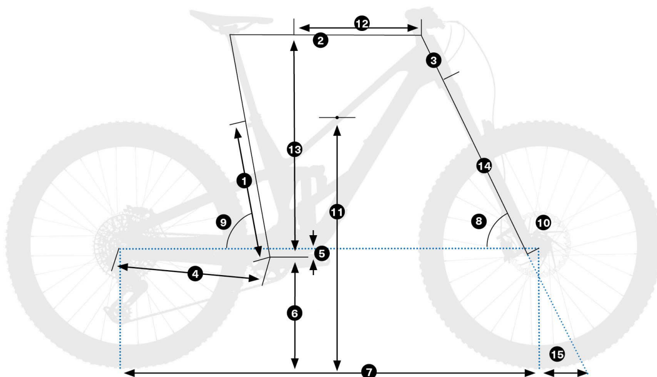
Orbea Rallon E-LTD 2026 – schemat geometrii ramy (źródło: Orbea)
