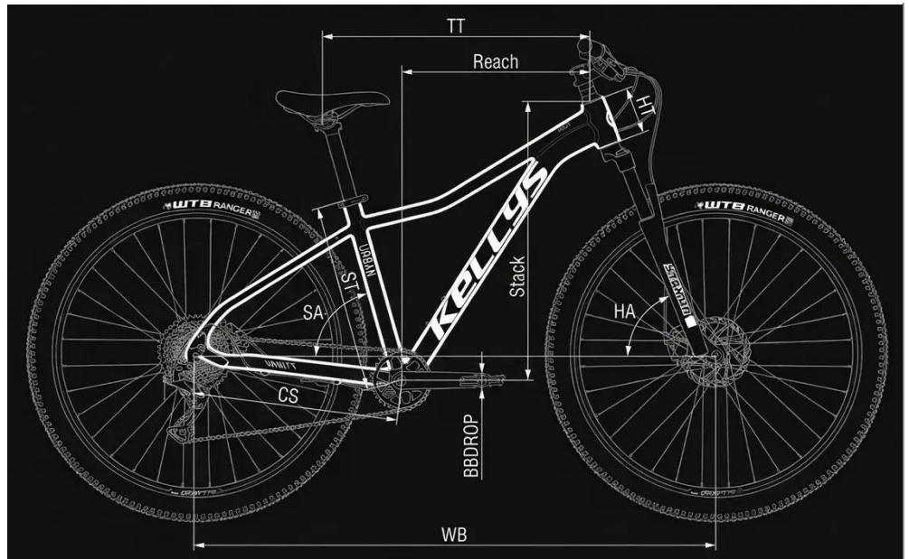
Schemat parametrów geometrycznych ramy VANITY
