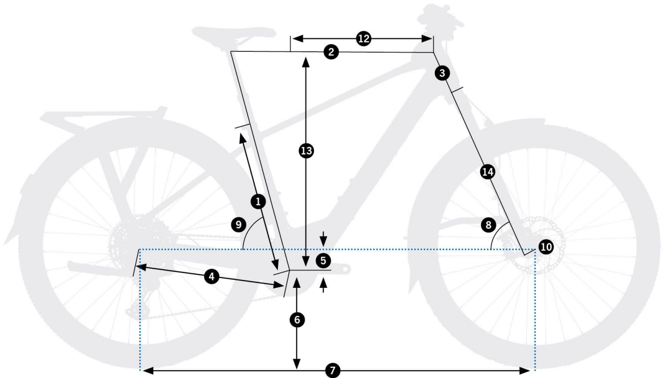
Schemat pomiarowy geometrii Orbea Kemen ADV 30 Mid
