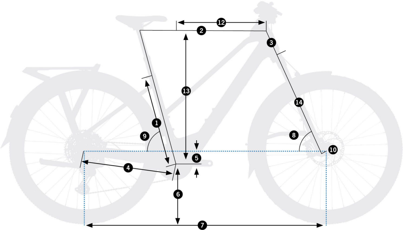
Schemat pomiarowy geometrii Orbea Kemen ADV 20 Mid
