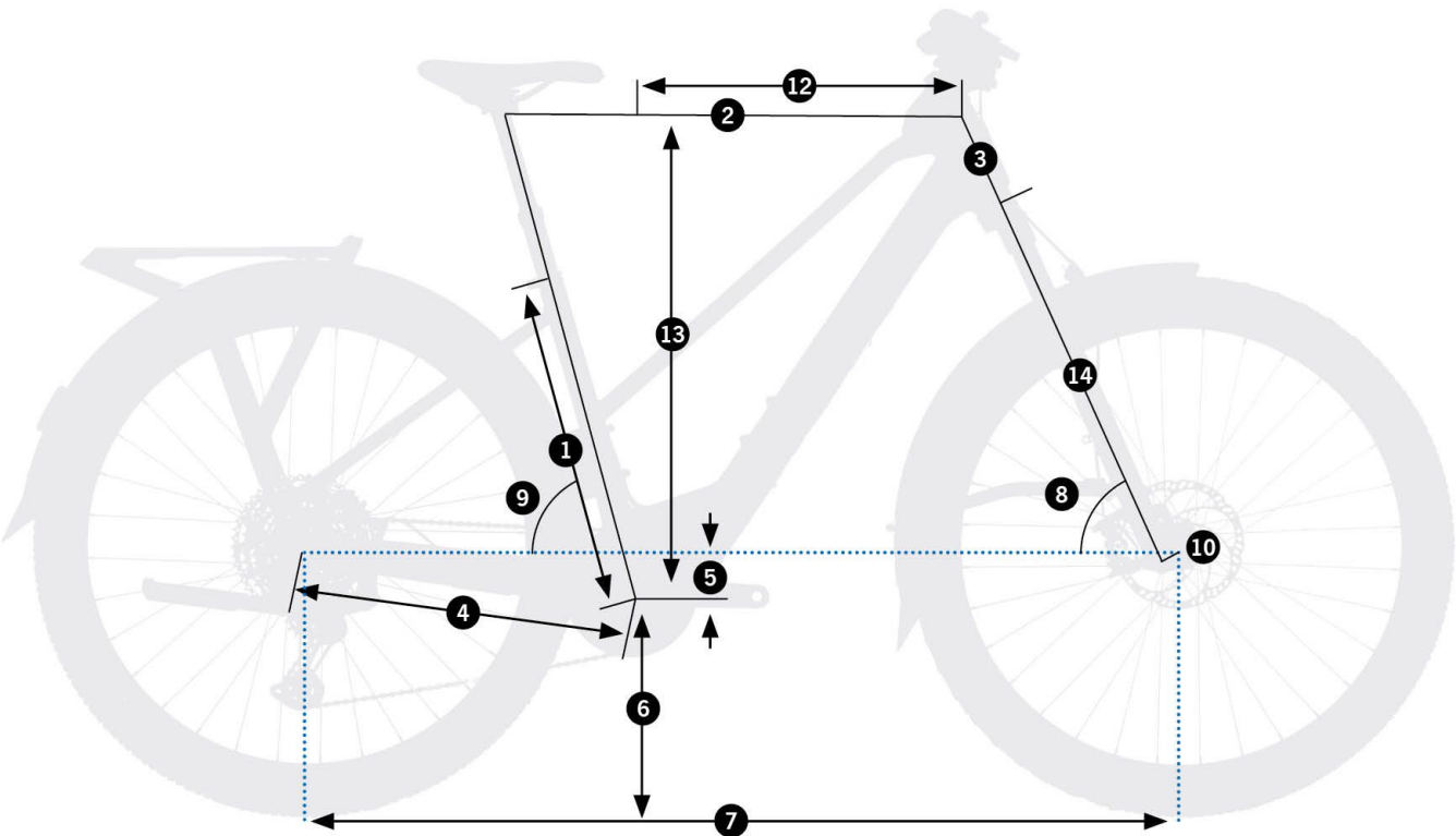
Schemat pomiarowy geometrii Orbea Kemen Tour 20 Mid
