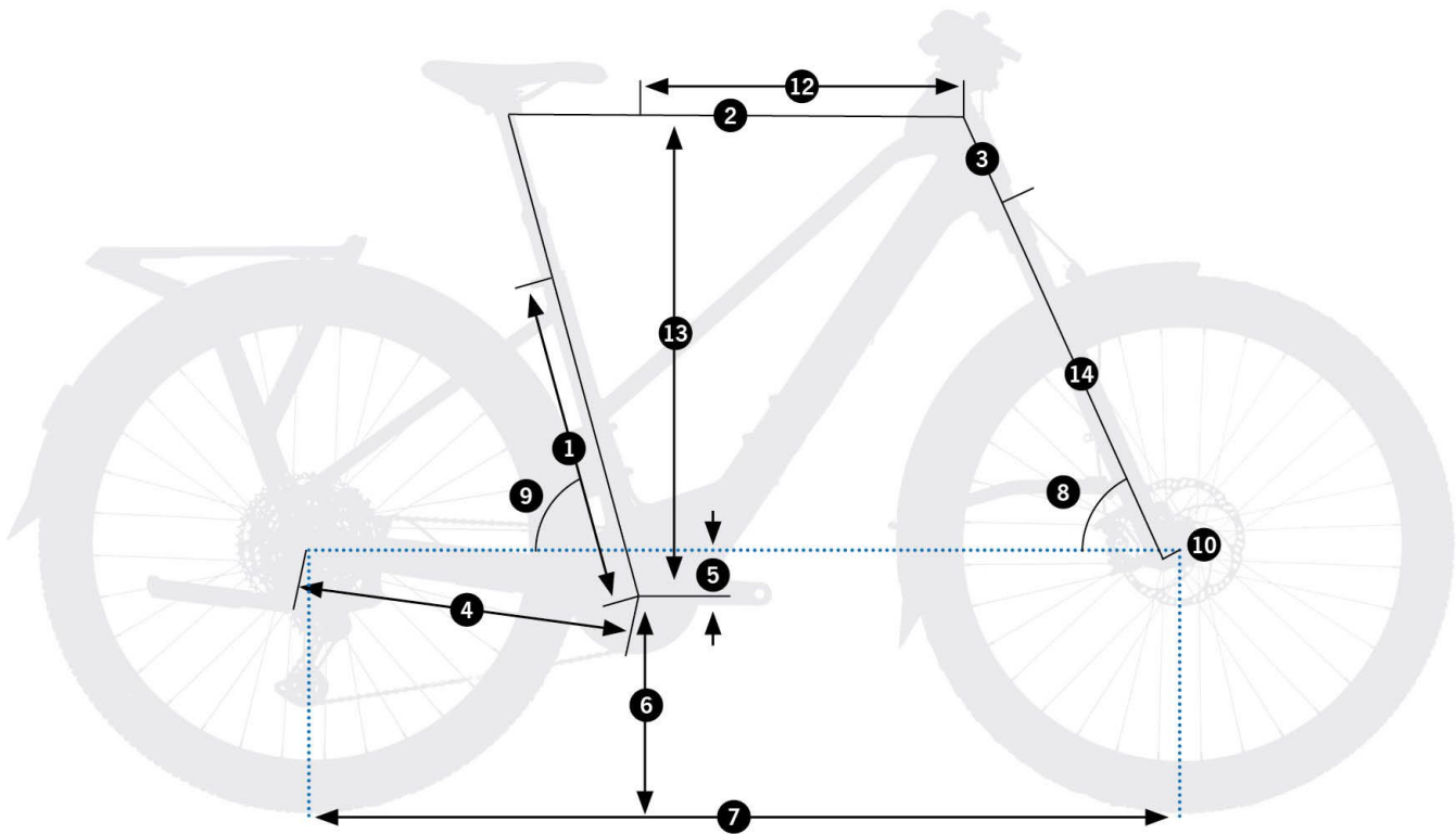
Schemat pomiarowy geometrii Orbea Kemen Tour 10 Mid
