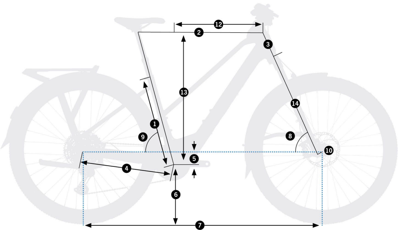
Schemat pomiarowy geometrii Orbea Kemen Tour 30 Mid
