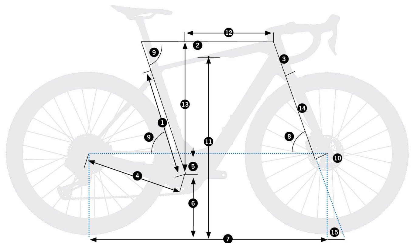
Orbea Denna M10i 2025 – schemat geometrii ramy (źródło: Orbea)
