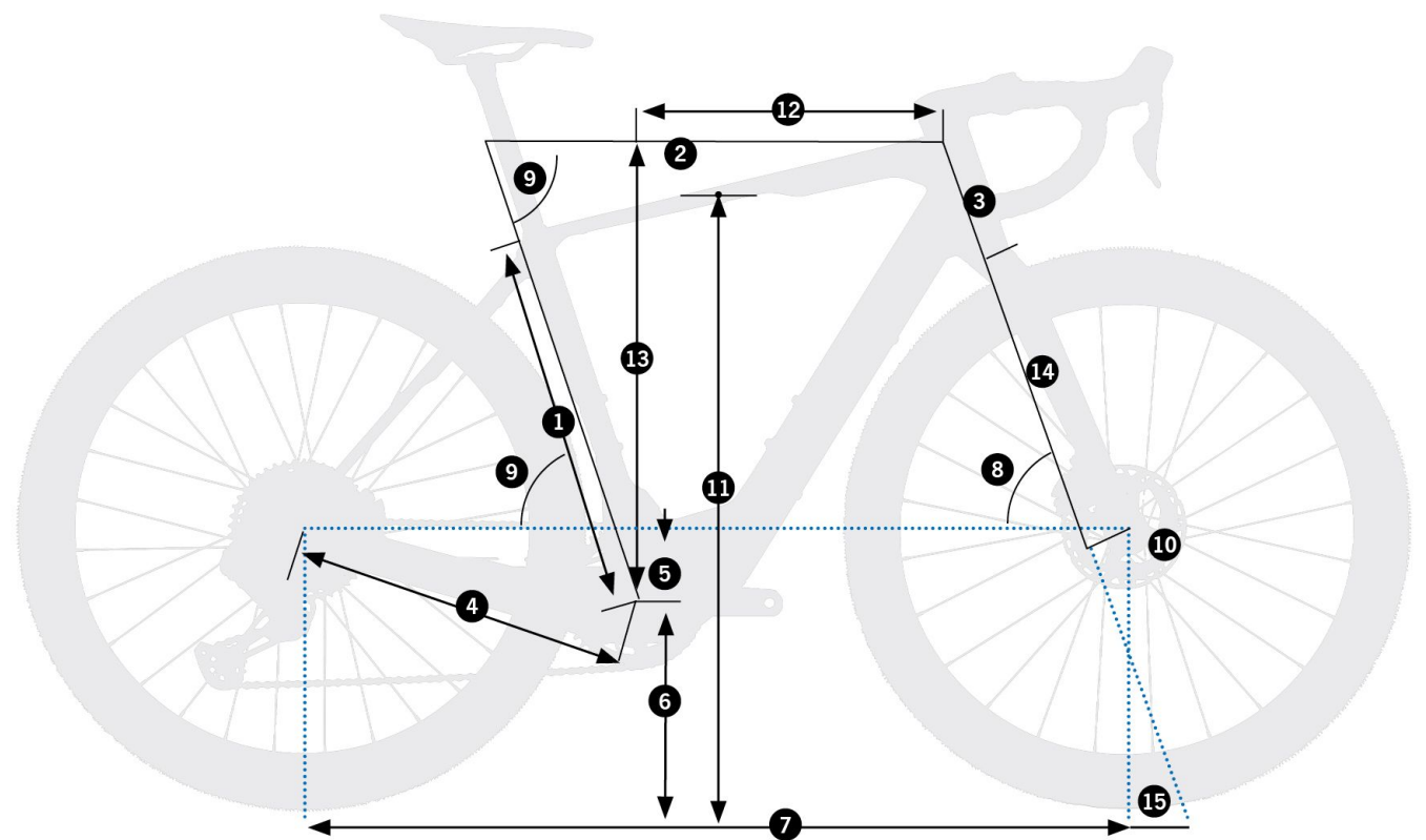
Orbea Denna H40 – schemat geometrii ramy (źródło: Orbea)
