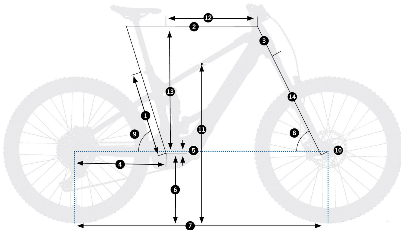
Schemat pomiarowy geometrii Wild M10
