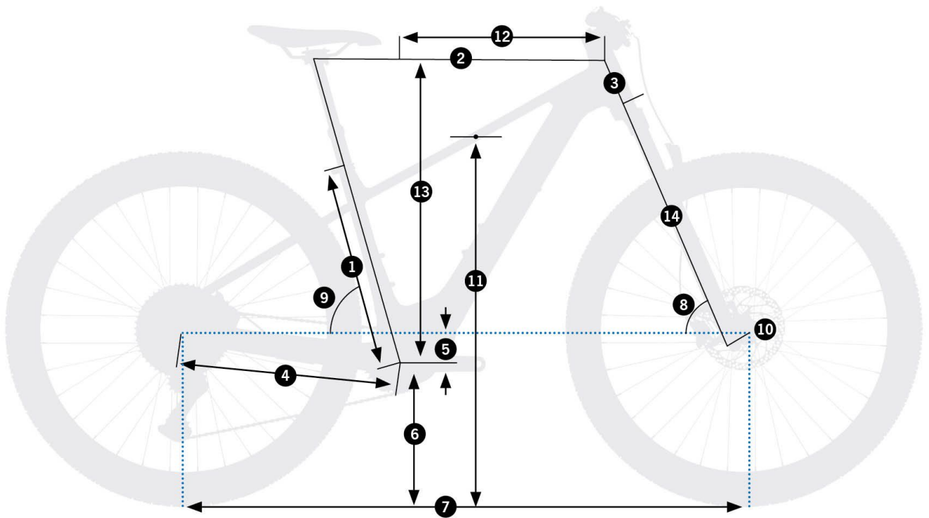
Orbea Urrun 30 2026 – schemat geometrii ramy (źródło: Orbea)
