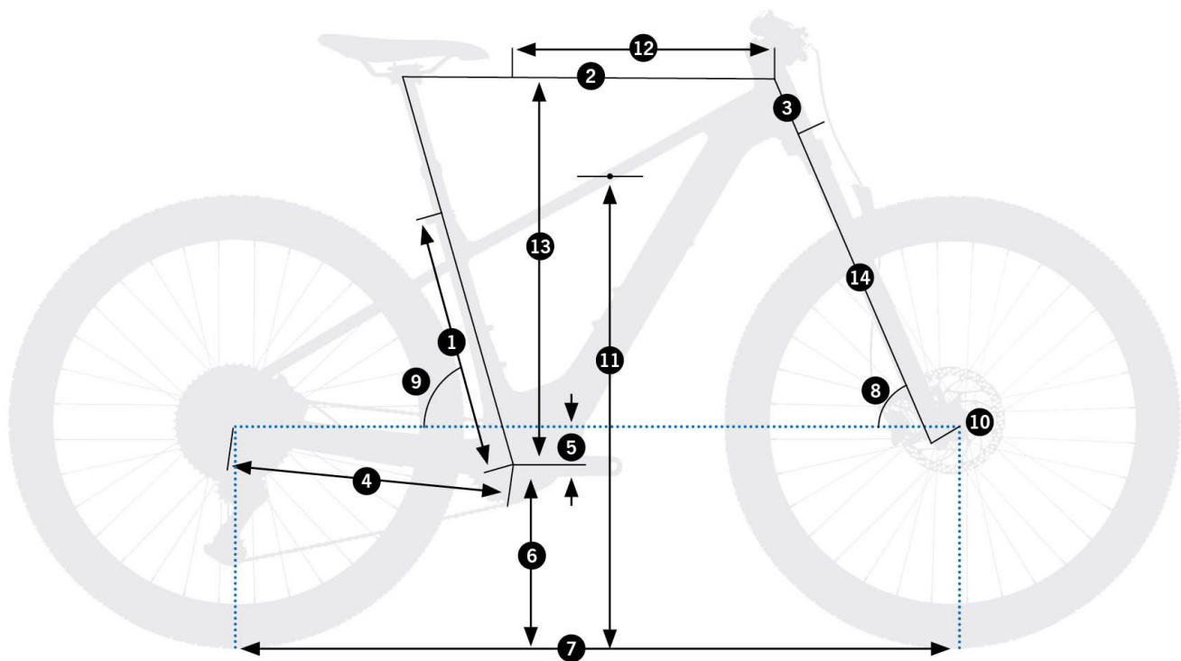
Orbea Urrun 20 2026 – schemat geometrii ramy (źródło: Orbea)
