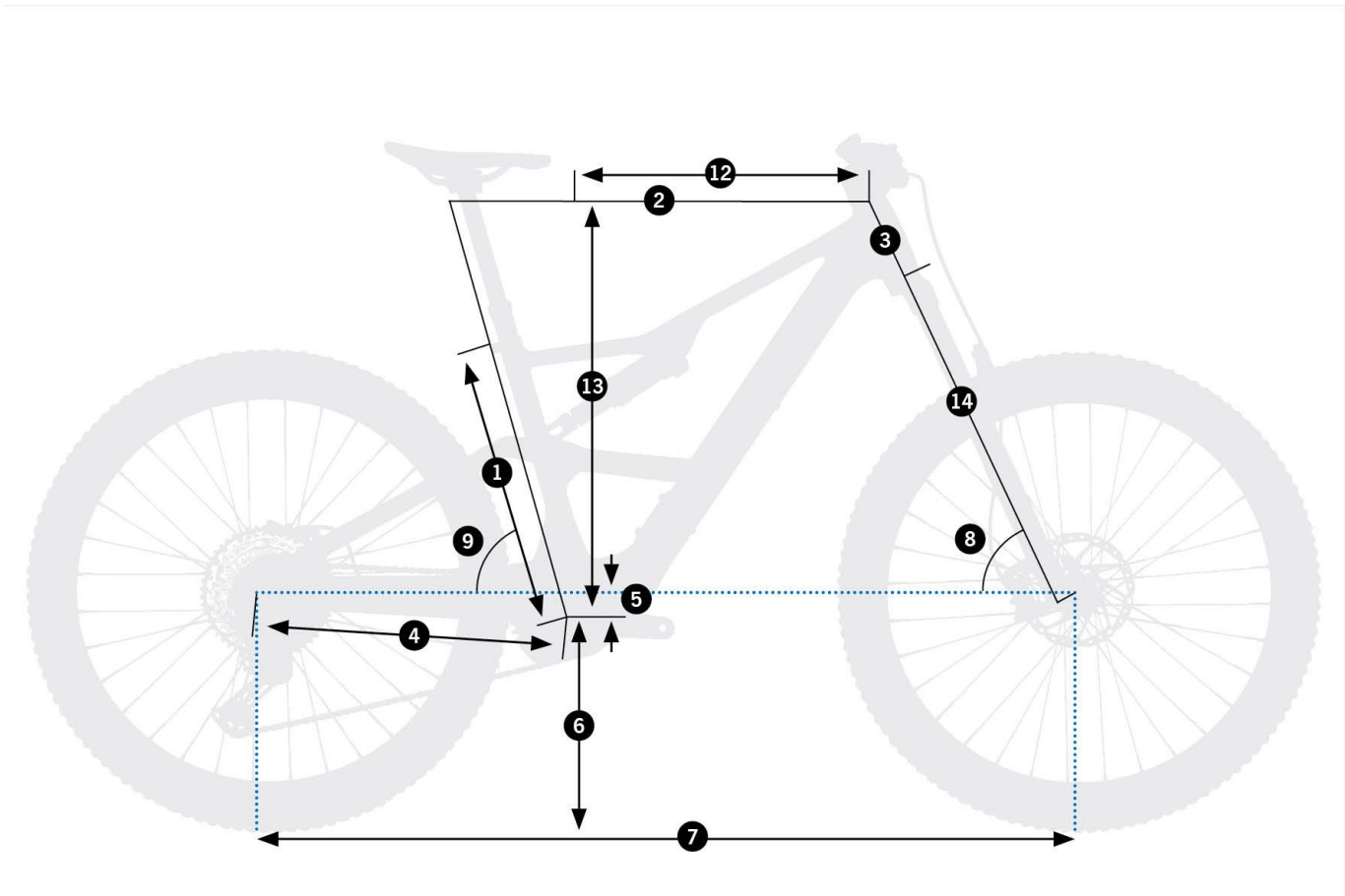
Orbea Rise SL H30 2026 – schemat geometrii ramy (źródło: Orbea)
