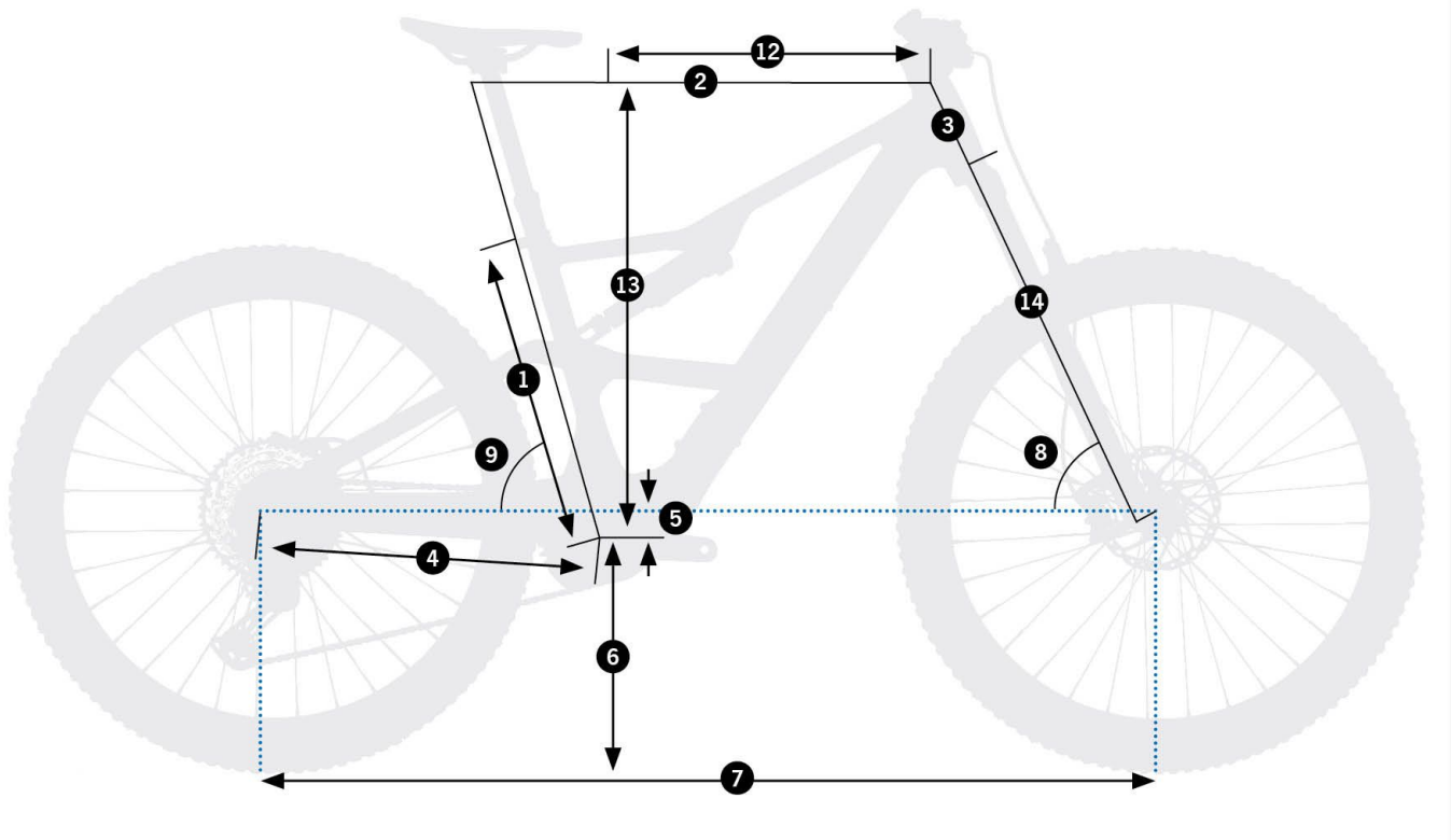
Orbea Rise SL H10 2026 – schemat geometrii ramy (źródło: Orbea)
