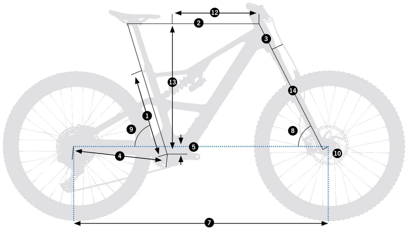
Rise LT M20 2026 - schemat geometrii ramy (źródło: Orbea)
