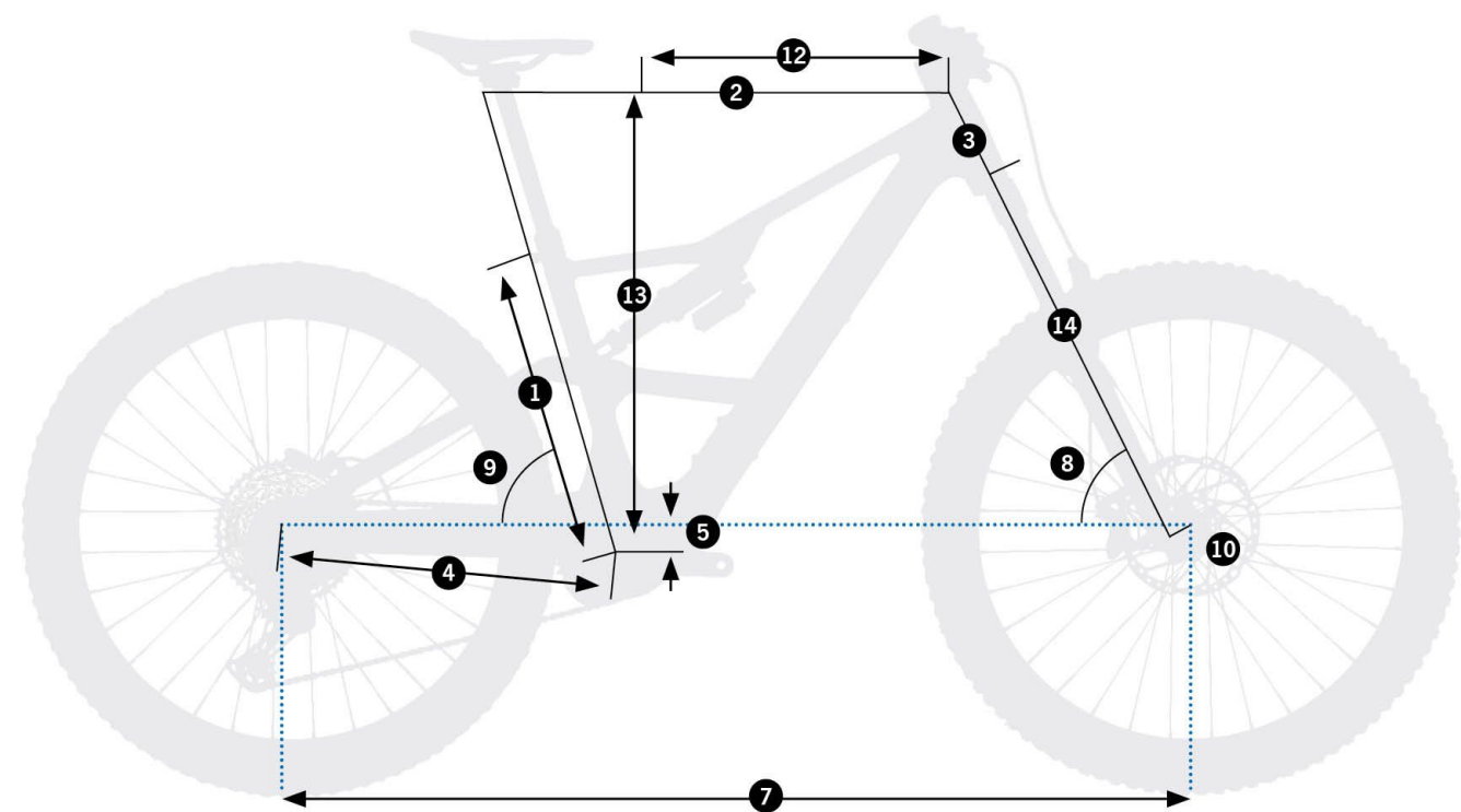
Rise LT H20 2026 – schemat geometrii ramy (źródło: Orbea)
