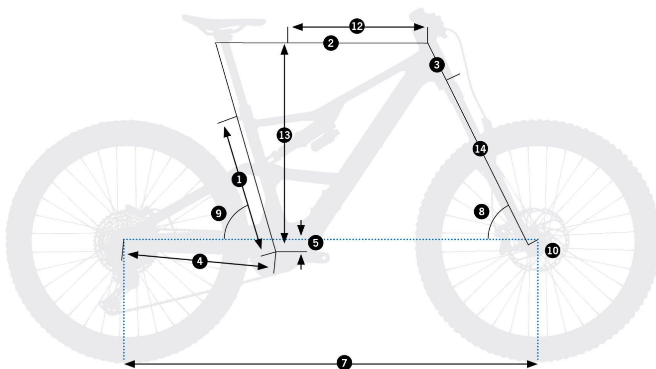
Rise LT H20 2026 - schemat geometrii ramy (źródło: Orbea)
