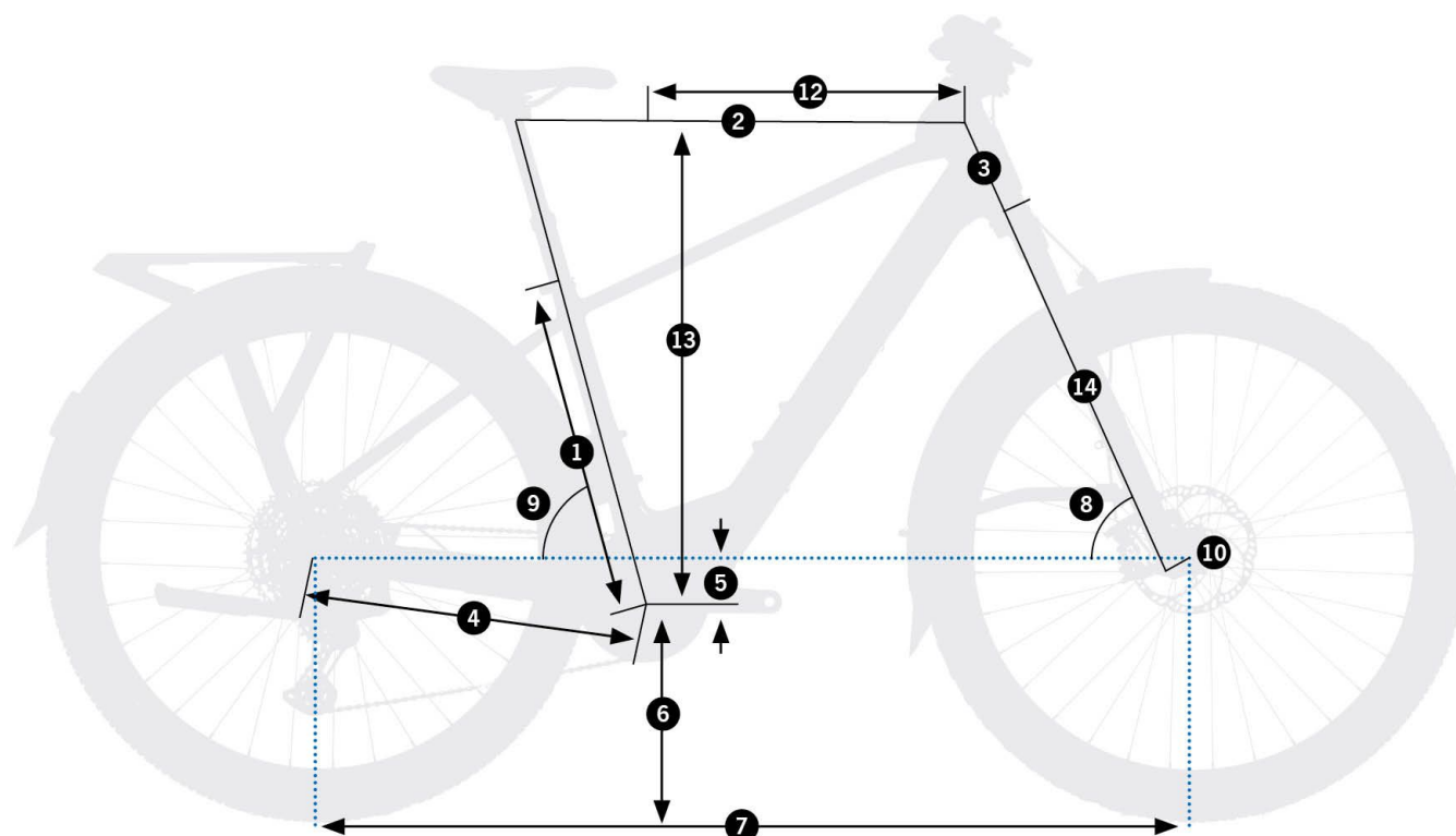
Schemat pomiarowy geometrii Orbea Kemen Tour 30
