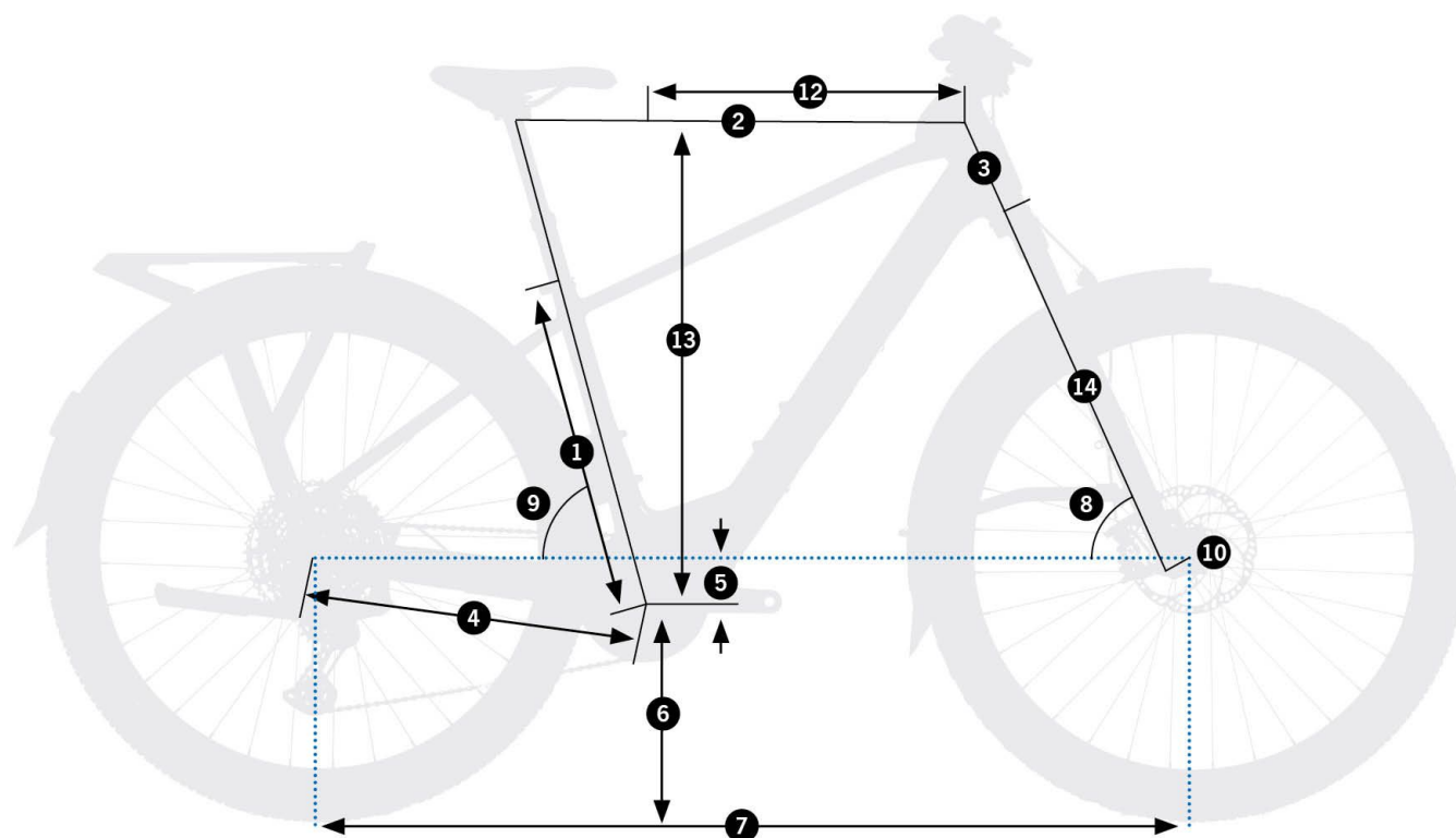
Schemat pomiarowy geometrii Orbea Kemen Tour 20
