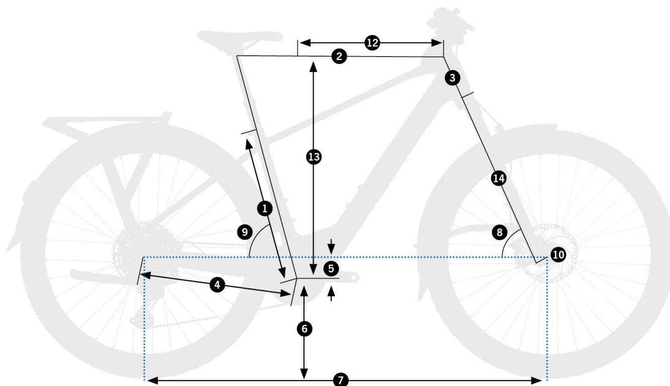
Schemat pomiarowy geometrii Orbea Kemen ADV 30
