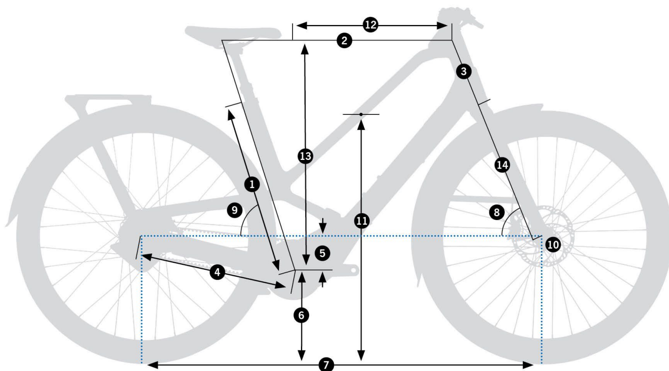
Schemat pomiarowy geometrii Orbea Diem 30
